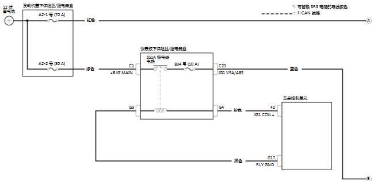
EPS 电路图
